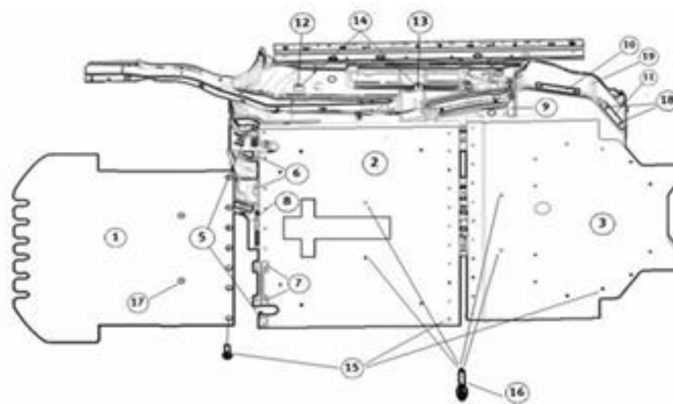
Рис. 8.3. Плоское дно.
