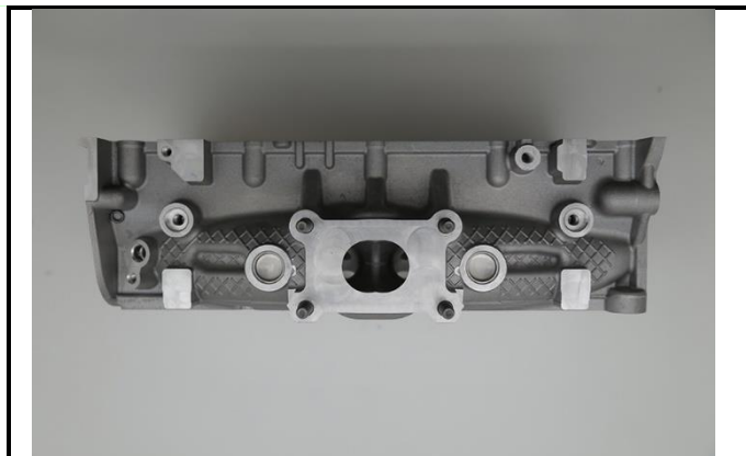
C8-4) Головка блока – вид со стороны выпуска
