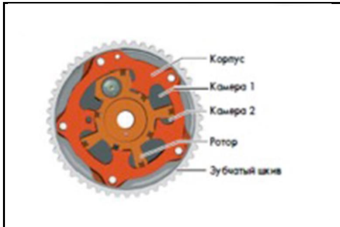
Устройство фазовариатора впускного распредвала /
